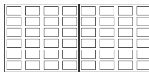
ref. P35N/308 42 x 23,5 x 2,5 cm
